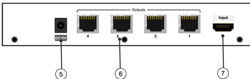
Achter paneel
