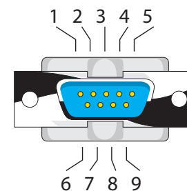
DB-9 (Male)
