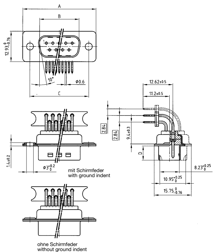
Stiftleiste / Plug connector
