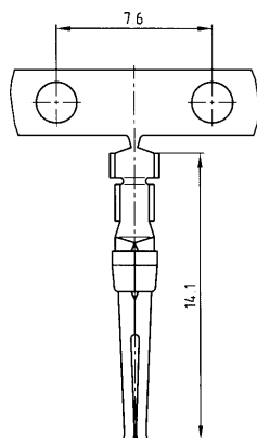
gestanzt stamped version
