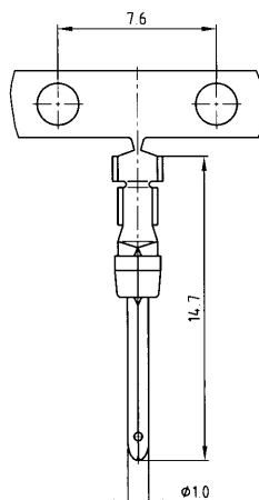
gestanzt stamped version
