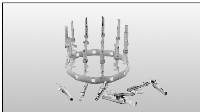
Crimp-Kontakte geeignet für Kabel AWG 24–20 und AWG 28–24
