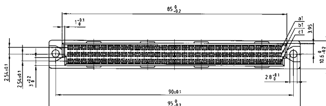
Wire Wrap
