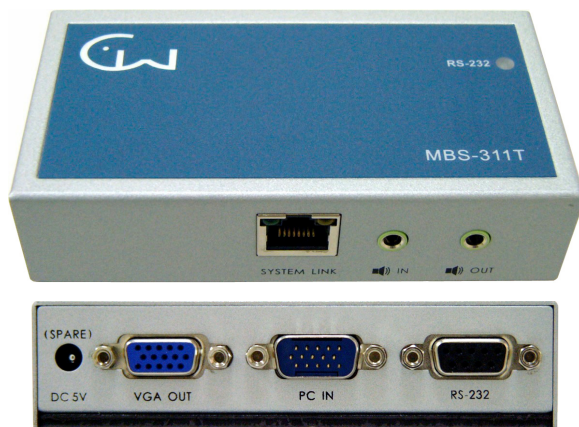
Transmitter(MBS-311T)
