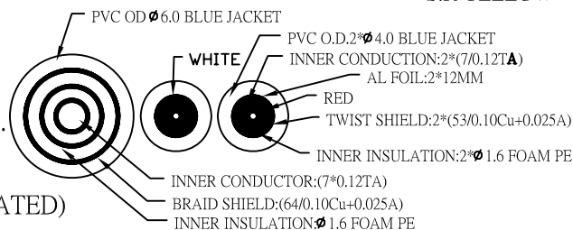
446-3C CABLE
